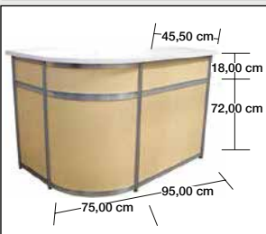
Διαστάσεις 1.00X3.00μ.
