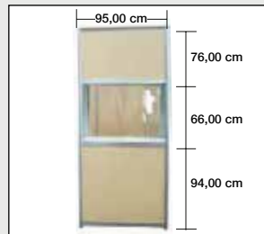
Διαστάσεις 1.00X2.50μ.
